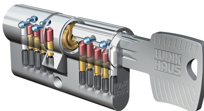
Abb.: 5-Stift-System
